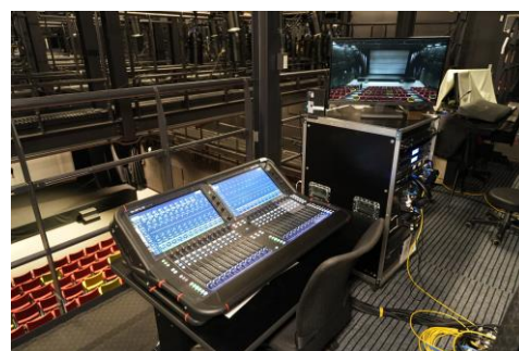
オーディオミキサー Allen &amp; Heath avantis
